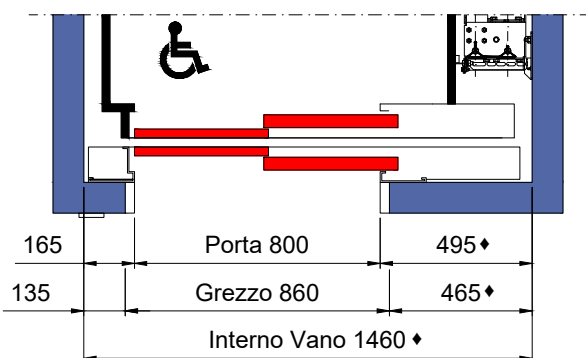
PIANTA VANO CORSA TELAIO PORTE NF (EI120)
