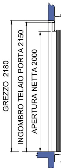
SEZIONE TELAIIO PORTE NF (EI120)
