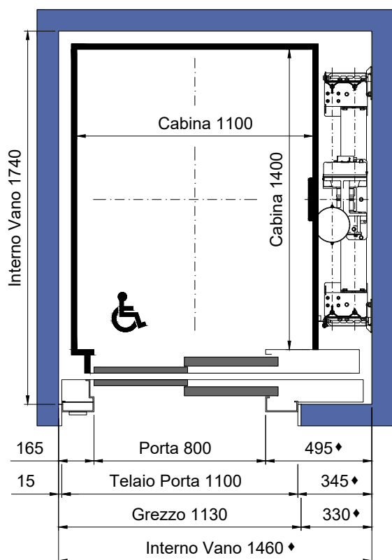
PIANTA VANO CORSA TELAIO PORTE MRF 150
