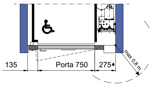
PIANTA PIANO GRUPPO DI MANOVRA TELAIO PORTE MRF 120 (STANDARD ED E120)
